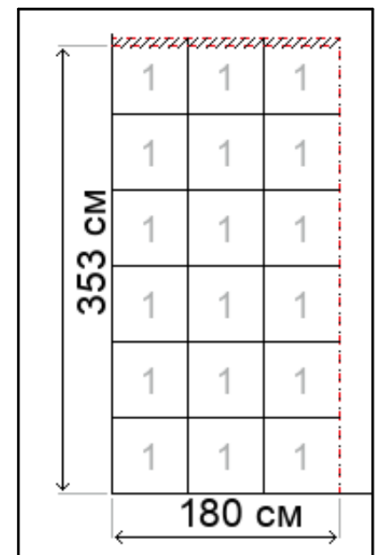
Схема монтажа гипсовых панелей
