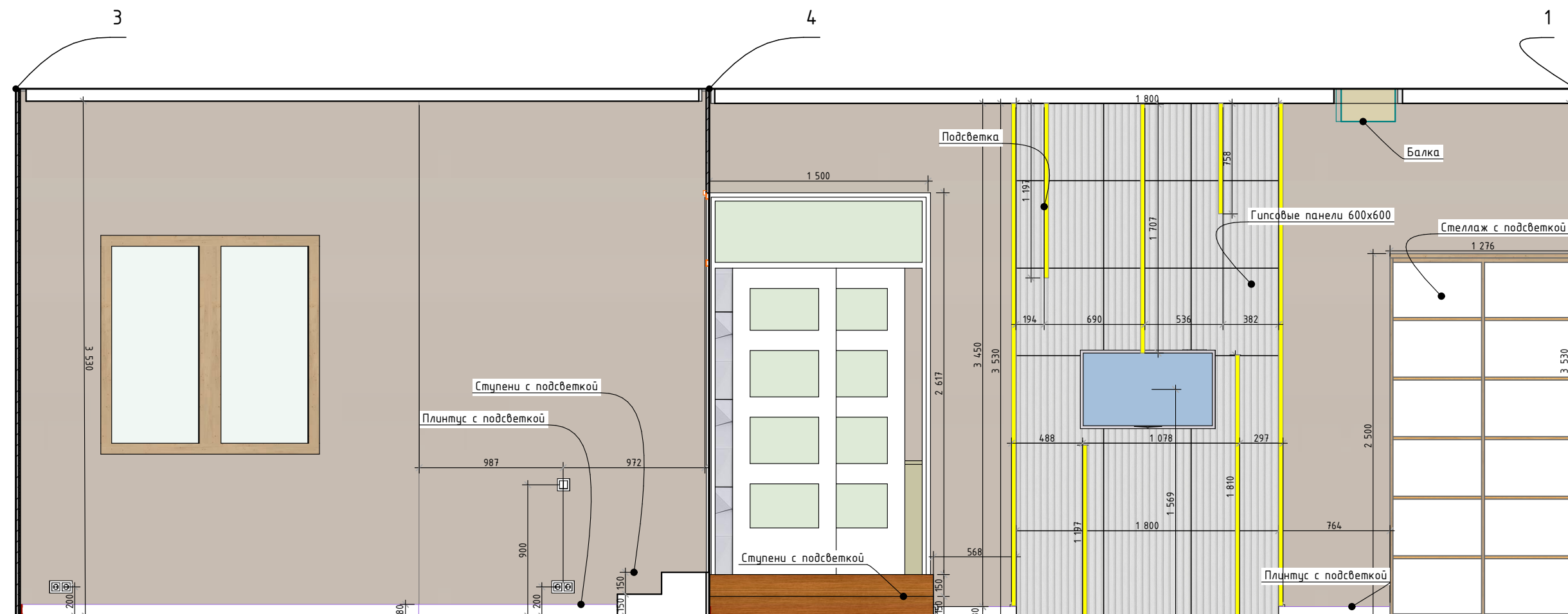
Схема монтажа гипсовых панелей
