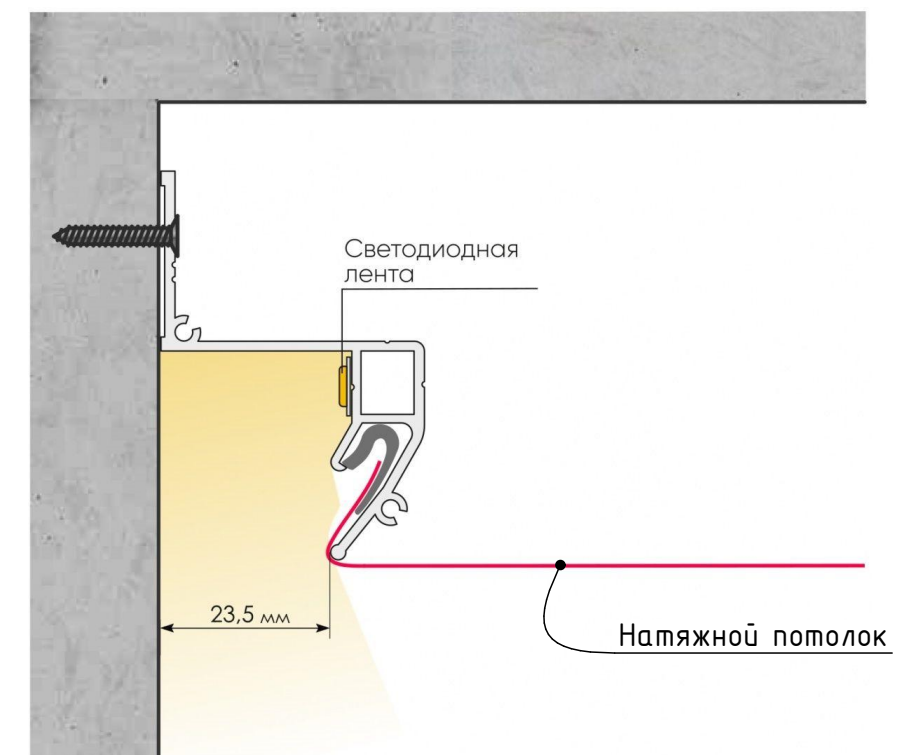
Вариант монтажа скрытой подсветки
